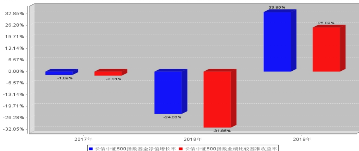
长信中证500指数自基金合同生效以来基金每年净值增长率及其与同期业绩比较基准收益率的对比图
