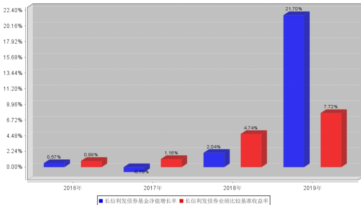
长信利发债券自基金合同生效以来基金每年净值增长率及其与同期业绩比较基准收益率的对比图
